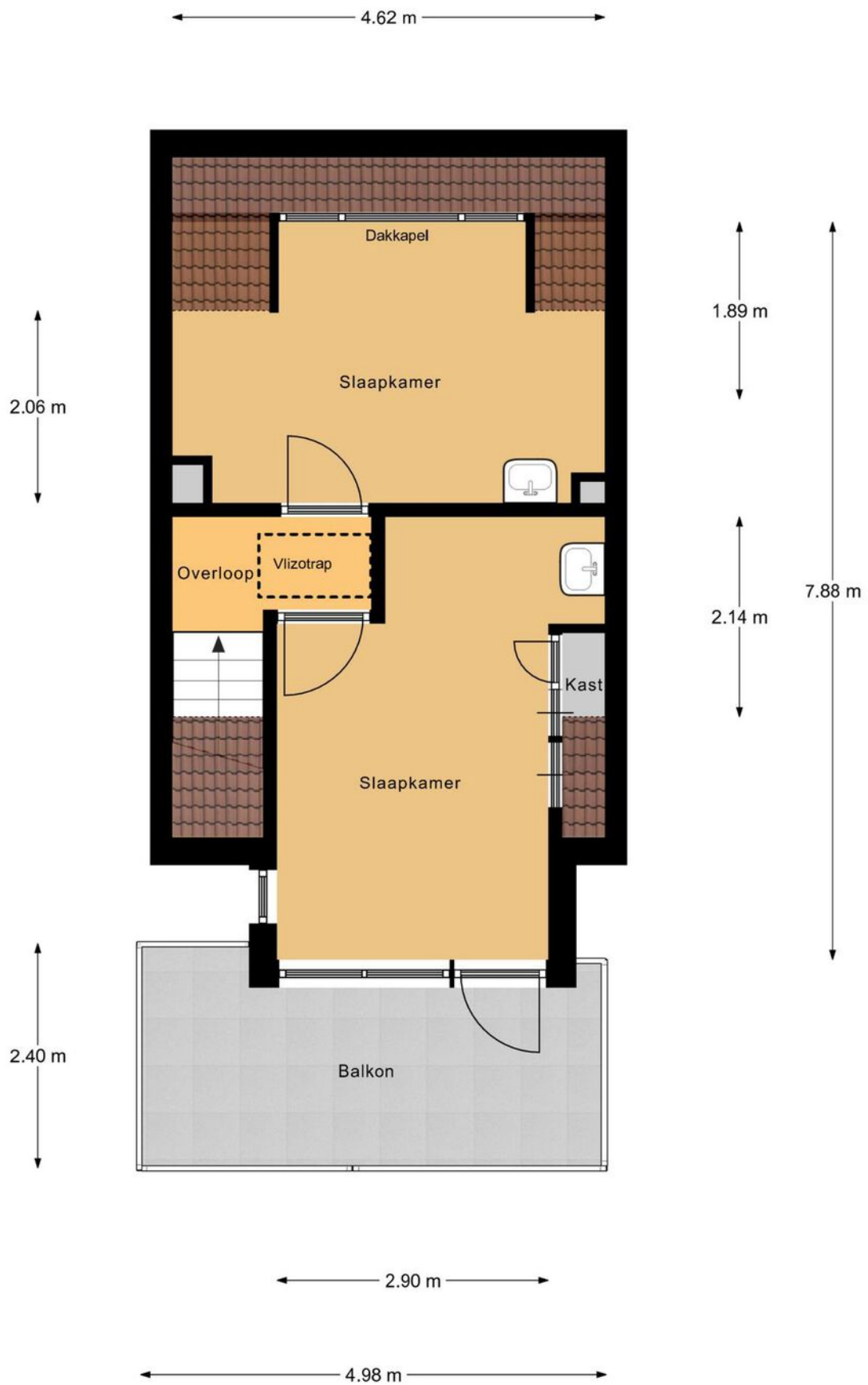
Tweede Verdieping
